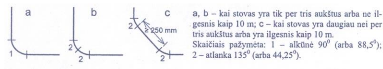
8.1 paveikslas. Stovo įjungimo į išvadą ar gulsčiąją dalį schemas
