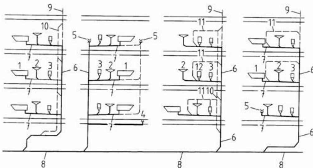
2 paveikslas. Nuotakyno (I ir II tipo sistemos) su vėdinimo stovais ir vėdinimo vamzdžiais schemų pavyzdžiai. Skaitiniai žymėjimai: 1 – vonia, 2 – praustuvas, 3 – išpuodis, 4 – trapas, 5 – orlaidis, 6 – stovas, 7 – nuotakas, 8 – išvadas, 9 – vėdinamoji stovo dalis, 10 – vėdinimo stovas, 11 – vėdinimo vamzdis, 12 – bidė.
