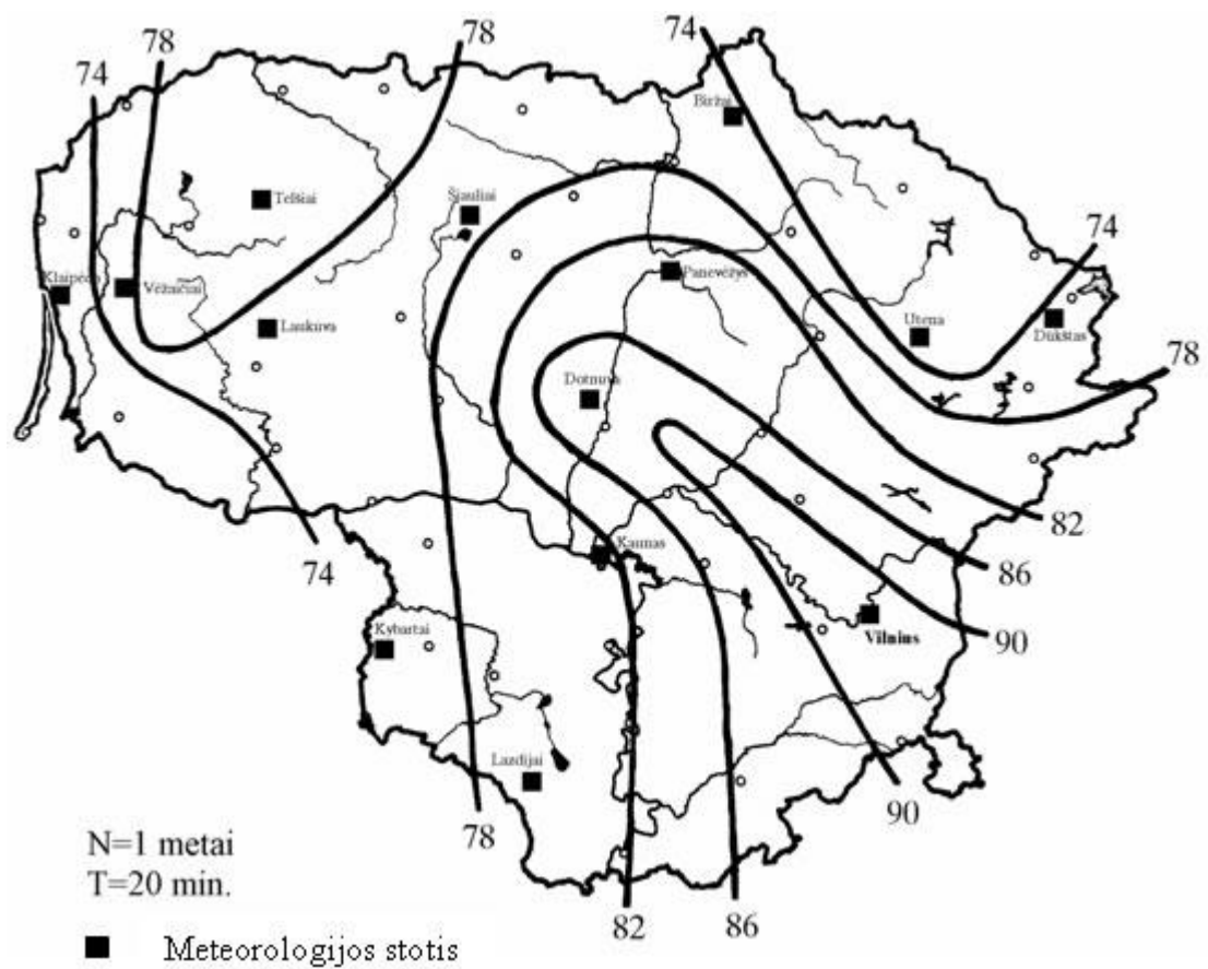
10.1 paveikslas. Kartą per metus pasikartojančio 20 minučių trukmės lietaus intensyvumo I/(sxha) pasiskirstymas Lietuvos Respublikoje
