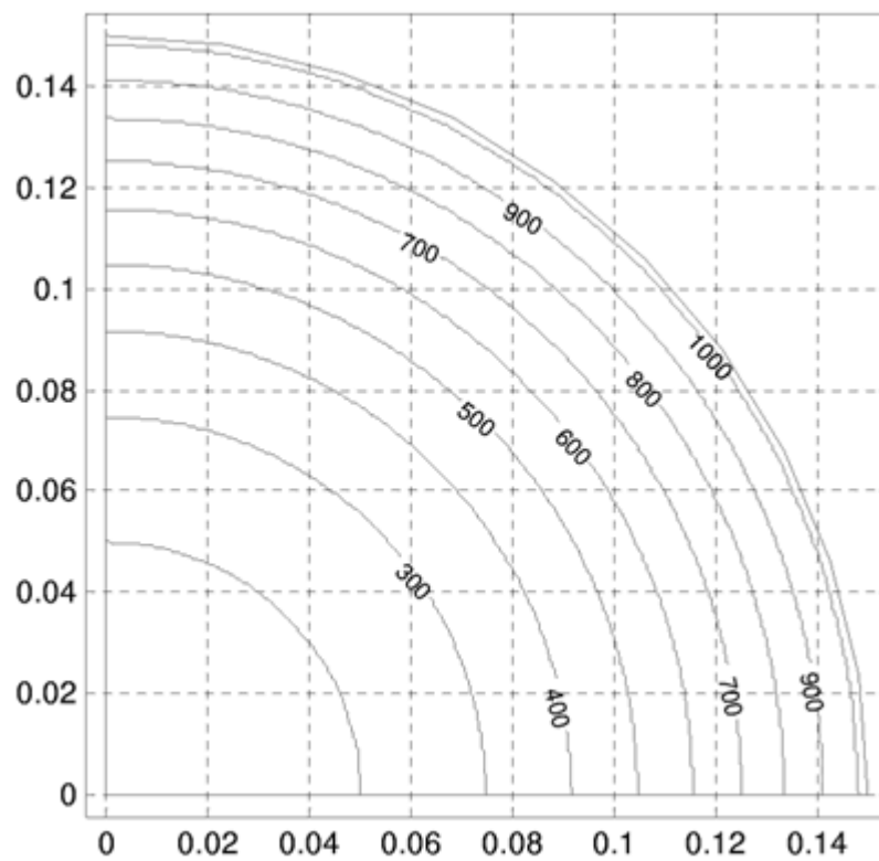
15 pav. Apvaliojo skerspjūvio kolonos, kurios \Delta E = 0,3 m ir R 120, temperatūrų laukai.
