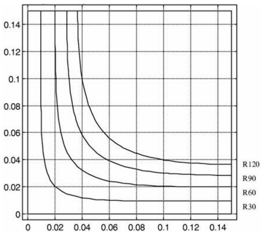
11 pav. Kolonos, kurios skerspjūvis h'b = 0,3'0,3 m, 500 °C izotermos.
