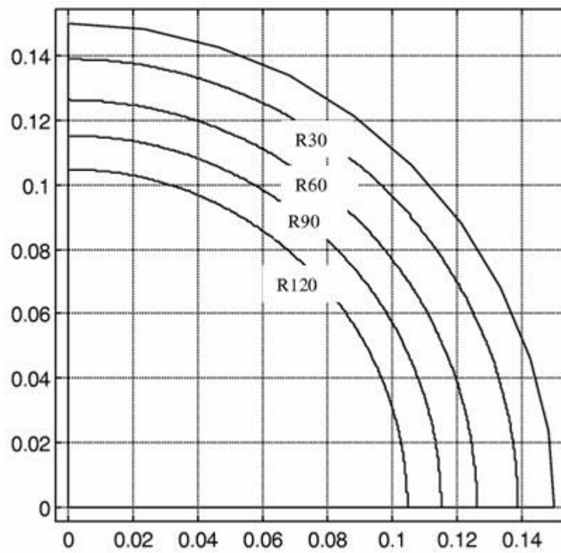
16 pav. Apvalaus skerspjūvio kolonos, kurios \lambda = 0,3 m, 500 °C izotermos.
