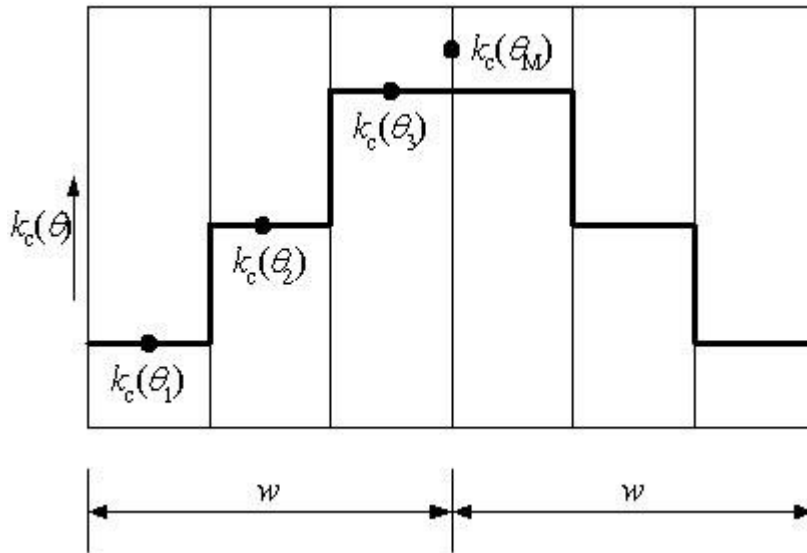
11 pav. Iš abiejų šonų gaisro veikiamos sienos ekvivalentinis suskirstymas į zonas betono stiprumo sumažinimo ir a_z reikšmės nustatymo tikslu.
