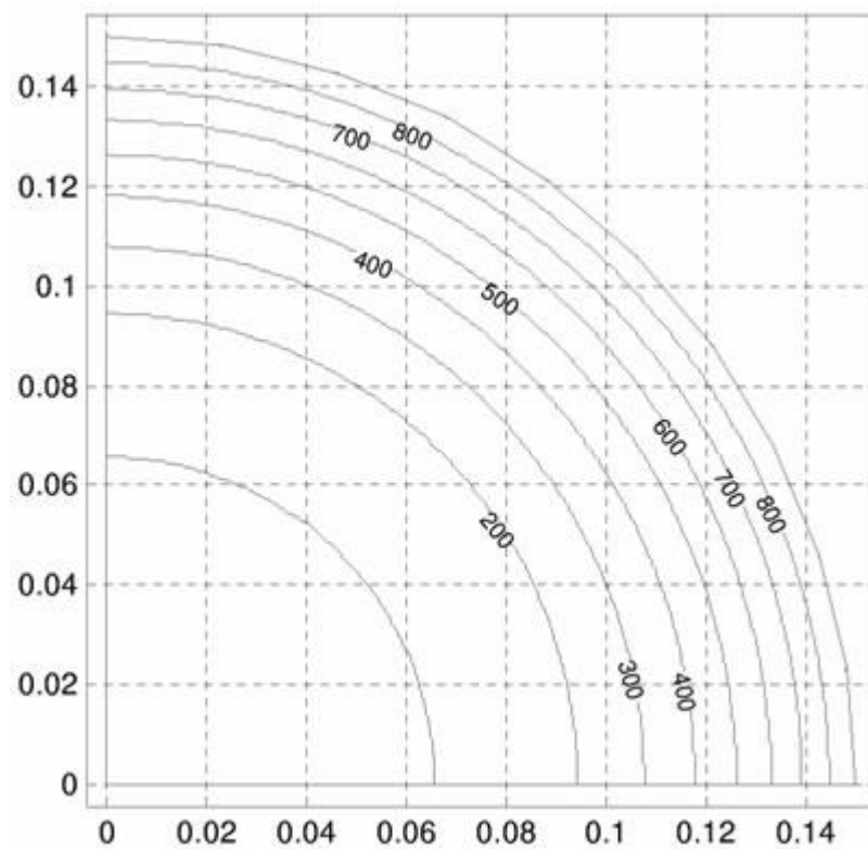
13 pav. Apvaliojo skerspjūvio kolonos, kurios \bar{A} = 0,3 m ir R 60, temperatūrų laukai.
