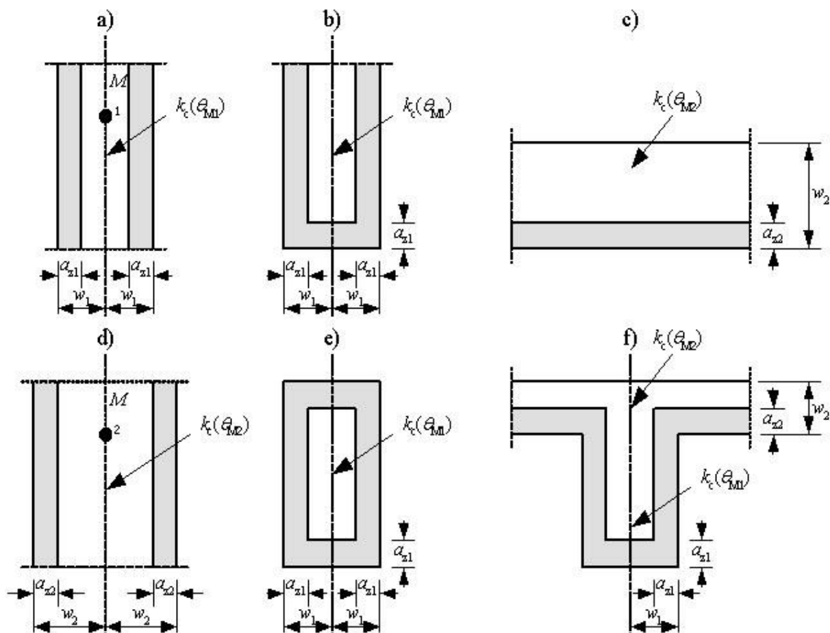
10 pav. Skerspjūvio ir betono stiprumo sumažinimo schemos.
