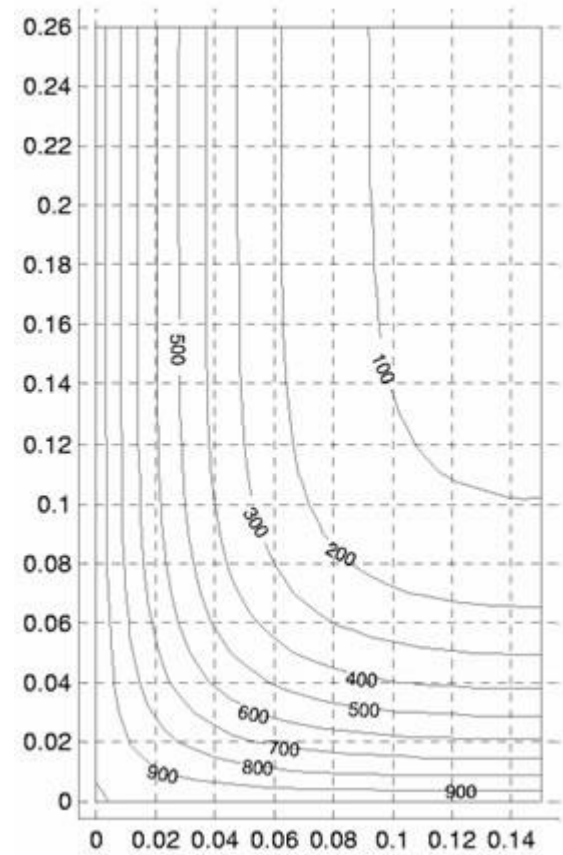
b) R 90
