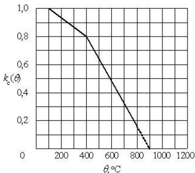
1 pav. Betono su granitiniais užpildais koeficiento k_c(q) priklausomybė nuo temperatūros.
