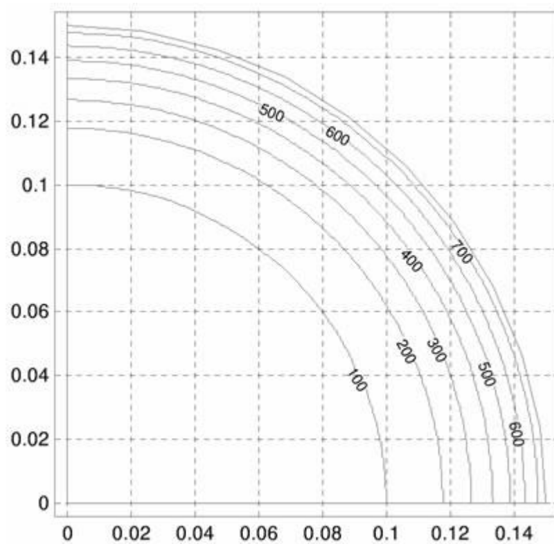
12 pav. Apvaliojo skerspjūvio kolonos, kurios \bar{A} = 0,3 m ir R 30, temperatūrų laukai.
