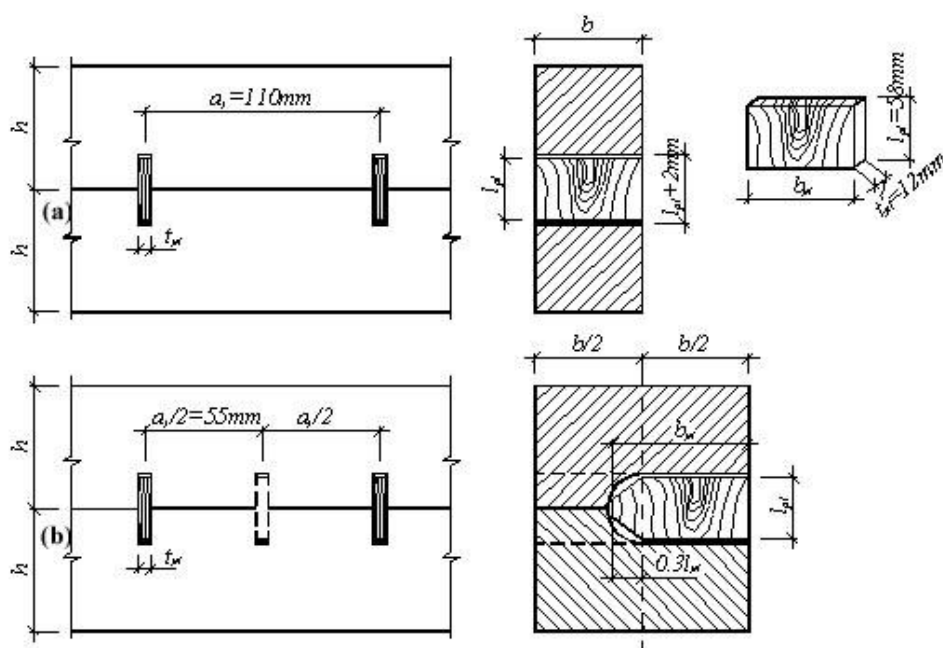
14 pav. Jungtys plokšteliniais kaiščiais: a – su kiaurai praeinančiu kaiščiu; b – su aklinuoju kaiščiu
