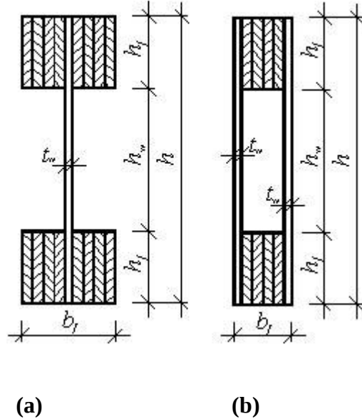
5 pav. Klijuotųjų sijų su plokščia fanerine sienie skerspjūviai: a – dvitėjinis; b – dėžinis
