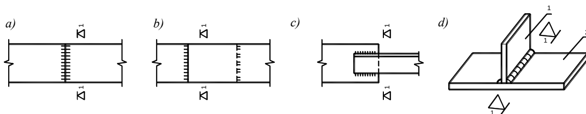
1 pav. Konstrukcijų virintinių jungčių schemas:
