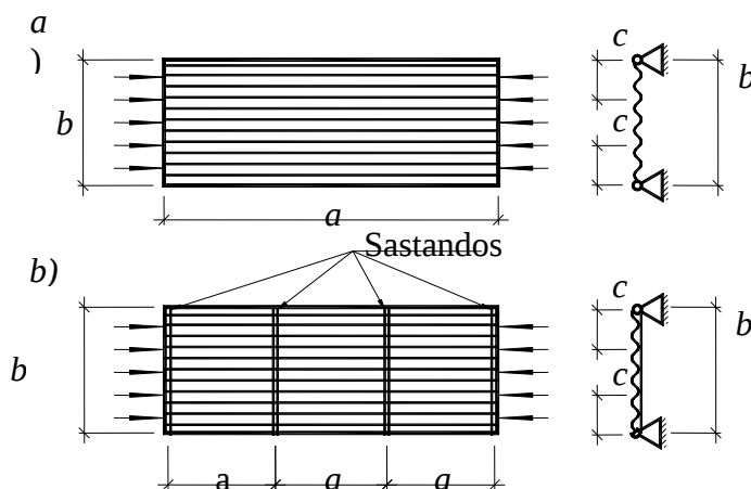
12 pav. Gniūždomojo gofruotojo lakšto skaičiuojamoji schema: a – kai nėra skersinių sąstandų; b – kai yra skersinės sąstandos
