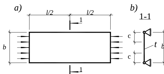
10 pav. Gniuždomojo plonalakščio elemento skaičiuojamoji schema: a – visas skerspjūvio plotis; b – veikiamasis skerspjūvio plotis
