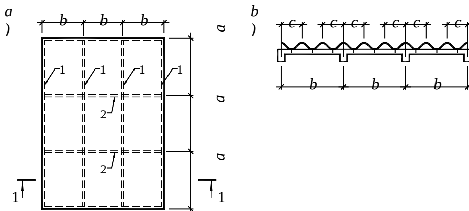
14 pav. Plokštės, kurią sudaro gofruotasis lakštas ir išilginės bei skersinės sąstandos, schema:
