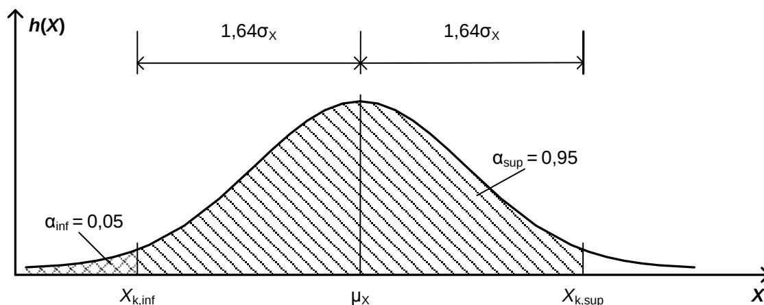
6 pav. Medžiagos ar grunto stiprio X minimali X_{k, \text{inf}} ir maksimali X_{k, \text{sup}} charakteristinės reikšmės; \alpha_{\text{inf}} = P(X < X_{k, \text{inf}}) = 0,05 ir \alpha_{\text{sup}} = P(X < X_{k, \text{sup}}) = 0,95 ; \mu_X ir \sigma_X – normalaus skirstinio tikimybės tankio h(X) vidurkis ir vidutinė kvadratinė nuokrypa
