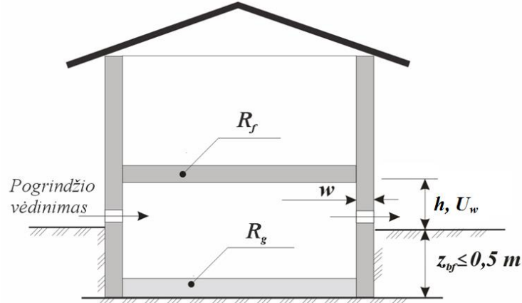
2.8. pav. Grindų virš vėdinamo pogrindžio schema
